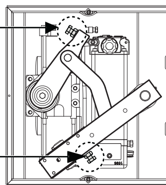
COMBI 787 AM RECHTEN TORFLÜGEL
