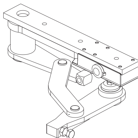
Detail des Hebels rechts Combi 787
