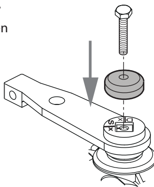
Bras de mouvement sur le Combi 787 gauche
