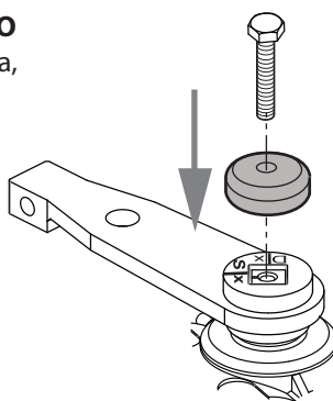
Braccio di movimento su Combi 787 sinistro
