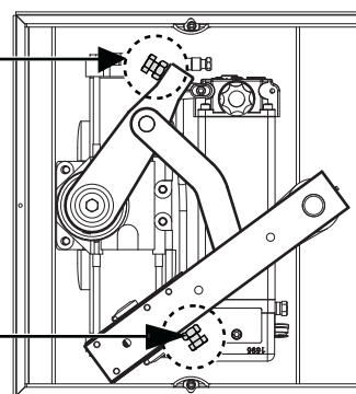
COMBI 787 SOBRE LA HOJA DERECHA
