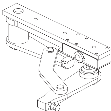
Particolare del levismo su Combi 787 destro
