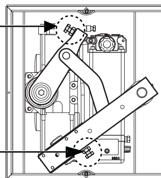
COMBI 787 SUR LE VANTAIL DROIT
