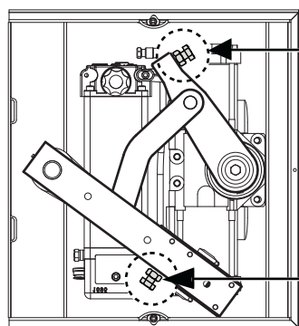
COMBI 787 SOBRE LA HOJA IZQUIERDA
