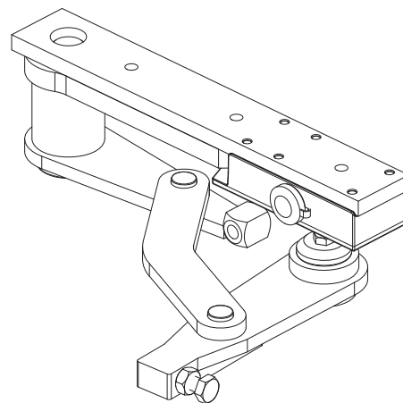
Détail du système de leviers sur le Combi 787 droite
