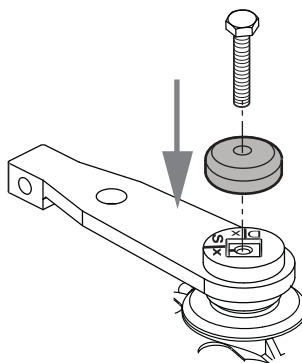
Brazo de movimiento sobre el Combi 787 izquierdo
