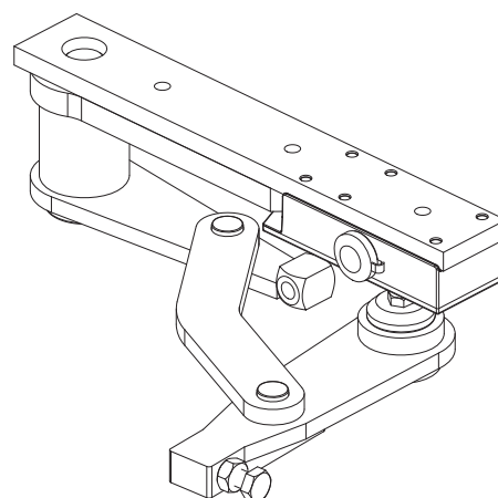
Particular de la biela sobre el Combi 787 derecho
